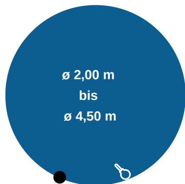
0,39 m Mitte Skimmer / Mitte Düse
